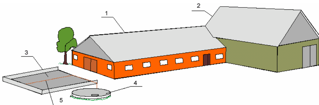
Figura 8.1 - Grajd cu așternut, capacitate pentru stocarea hranei, groapă de gunoi și rezervor pentru stocarea urinei. 1: grajd, 2: incintă pentru stocarea furajrlor, 3: platformă , 4: rezervor pentru mustul de gunoi, 5: canale pentru scurgerea mustului de gunoi. (preluată după Codul de Bune Practici Agricole elaborat de Lituania)
