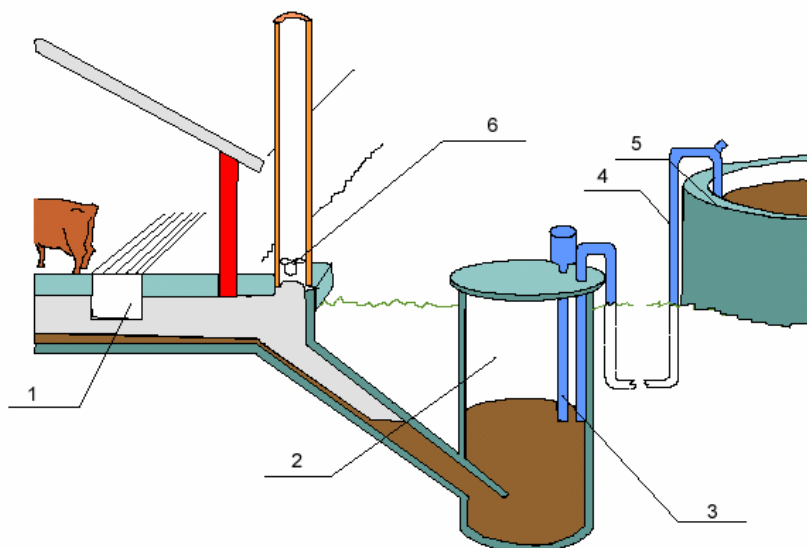
Figura 8.3 - Exemplu de sistem pentru eliminarea dejectiilor lichide 1 : canal pentru scurgerea dejectiilor lichide, 2 : fosa pentru stocarea intermediara a dejectiilor lichide, 3 : pompa, 4 : tuburi, 5 : rezervor pentru stocarea dejectiilor lichide, 6 : ventilatie (preluata dupa Codul de Bune Practici Agricole elaborat de Lituania)
