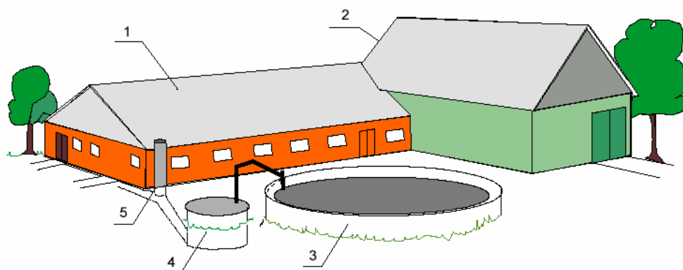
Figura 8.2 - Grajd fără asternut. 1: grajd, 2: incintă pentru stocarea furajelor, 3: rezervor pentru depozitarea temporară a deșeurilor fluide, 4: fosă pentru colectarea deșeurilor fluide, 5: tub de ventilație (preluată după Codul de Bune Practici Agricole elaborat de Lituania)
